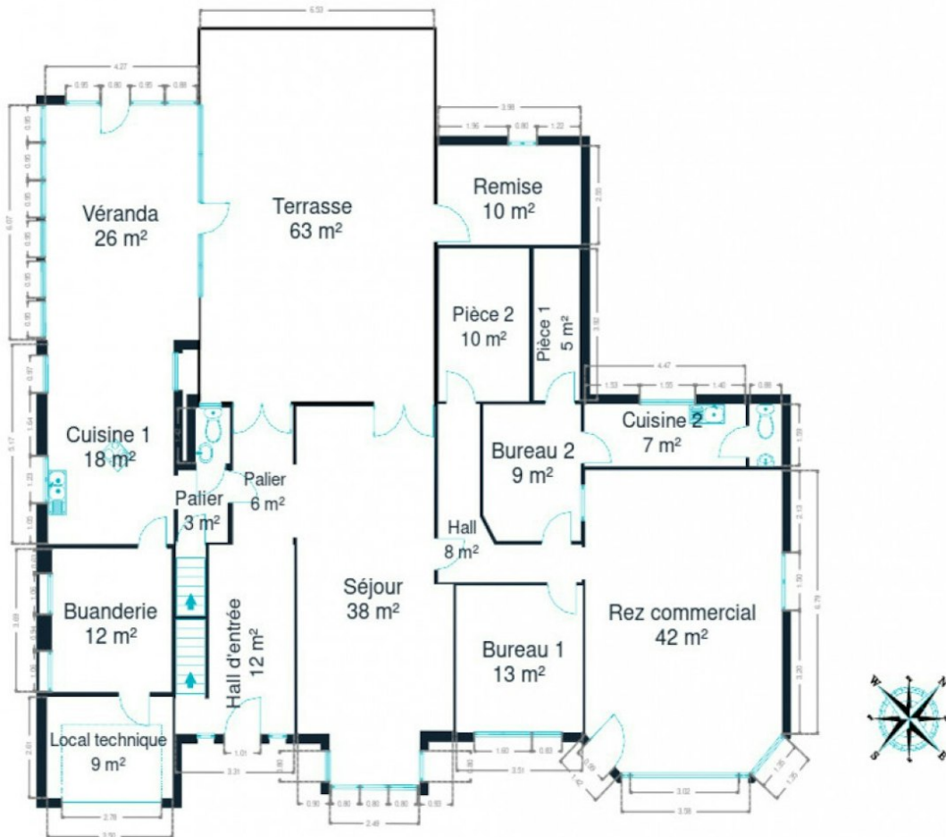
Rez-de-chaussée
